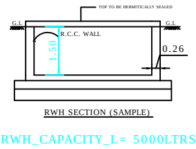
RWV_CAPACITY_L= 5000LTRS
