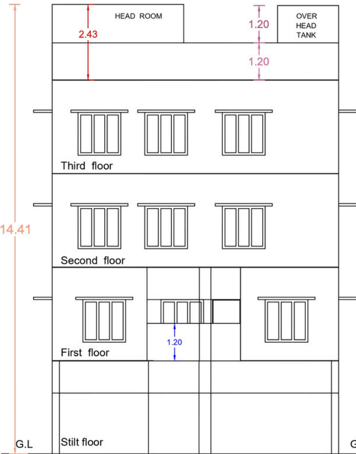
ELEVATION
