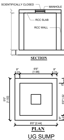
UG SUMP
