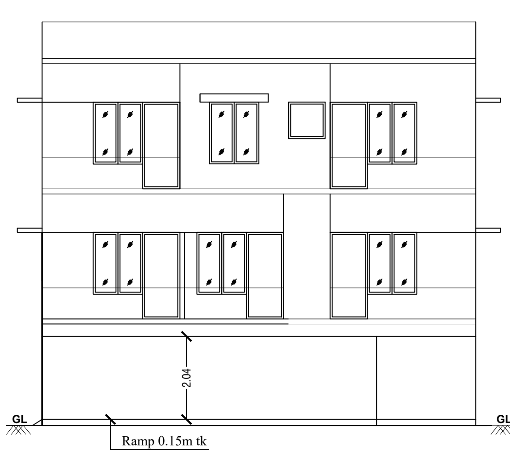
ELEVATION
