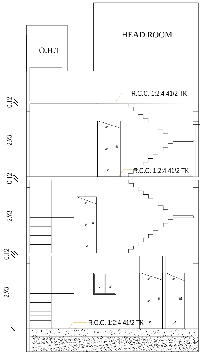
SECTION -AB
