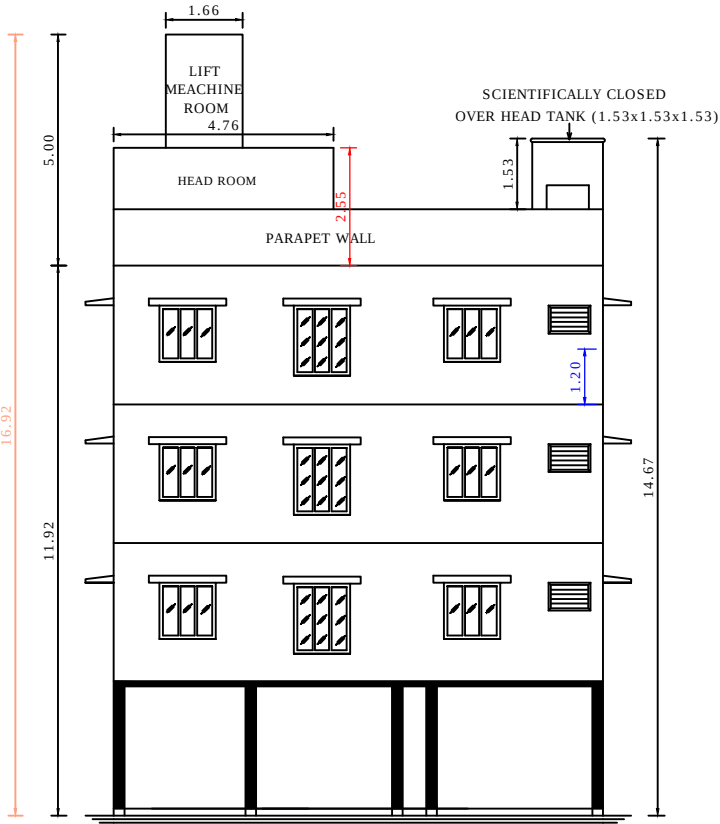
ELEVATION
