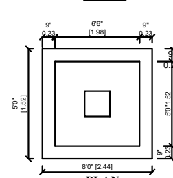
UG SUMP
