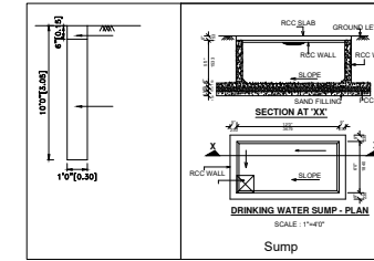
Sump
