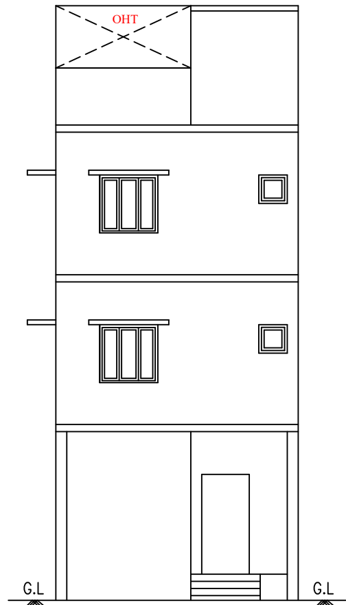
ELEVATION
