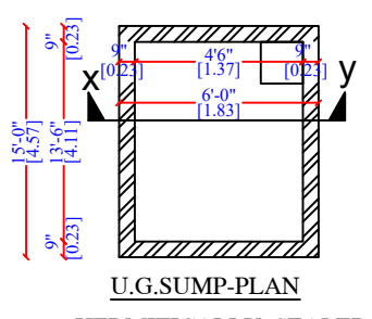
U.G. SUMP-PLAN
