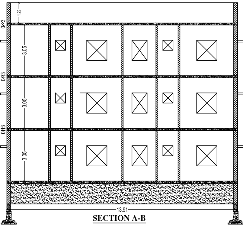
SECTION A-B
