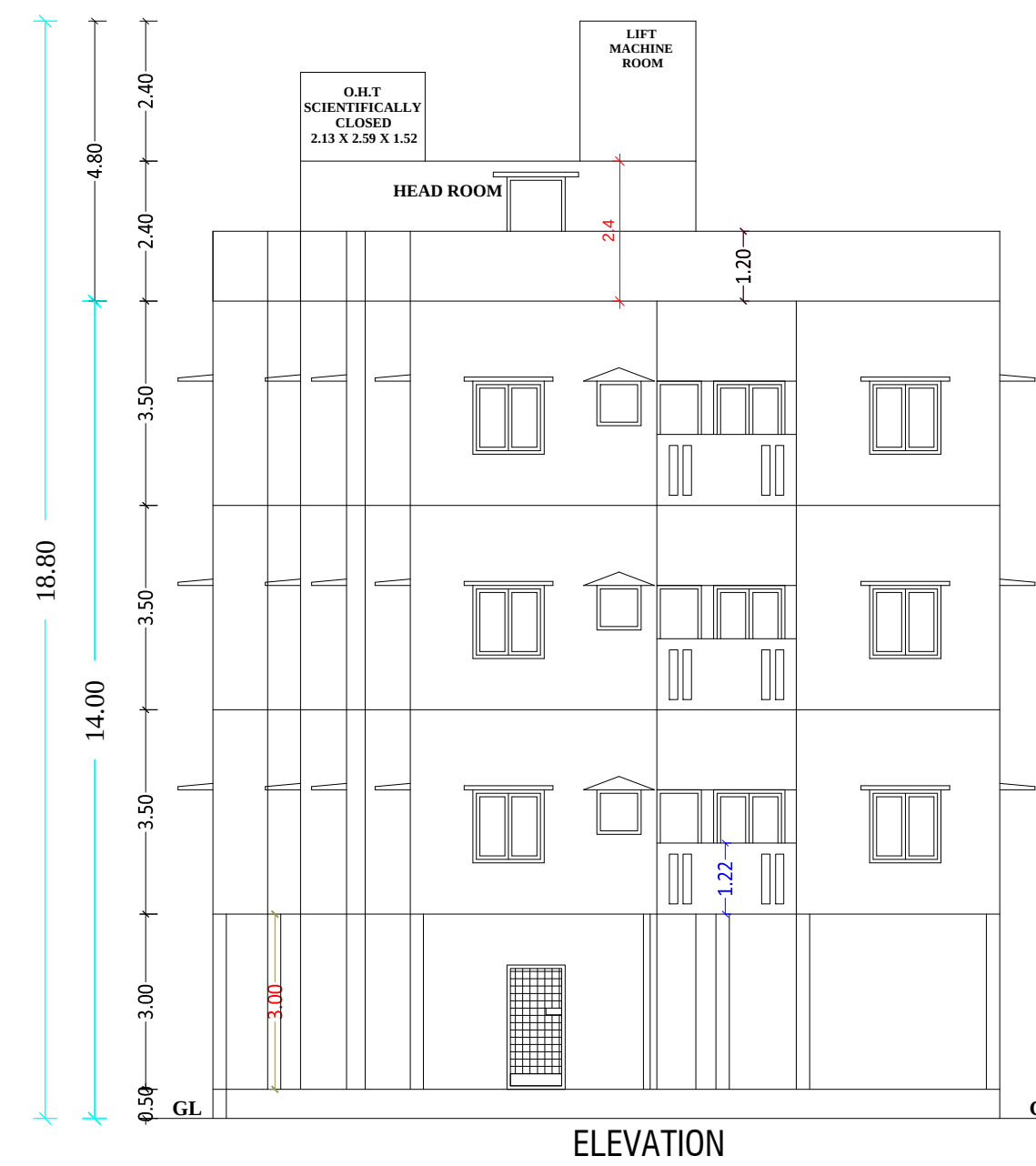
ELEVATION
