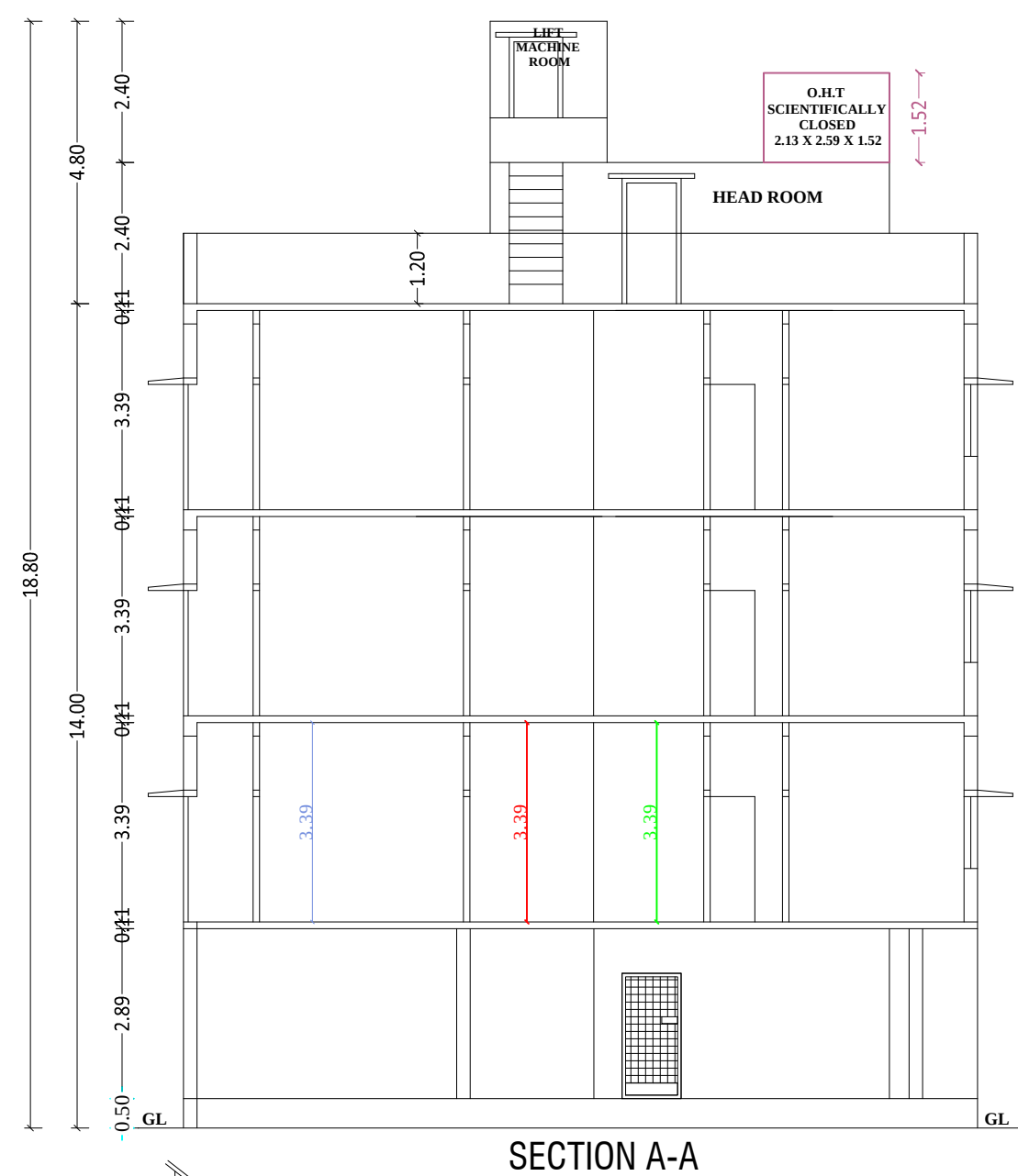
SECTION A-A
