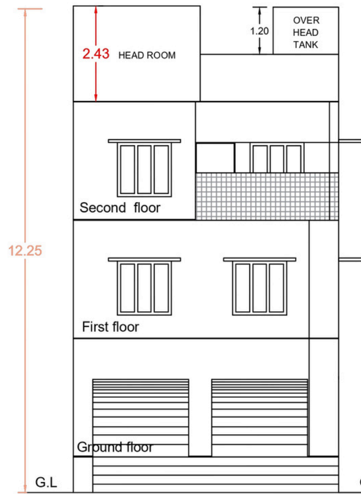
ELEVATION
