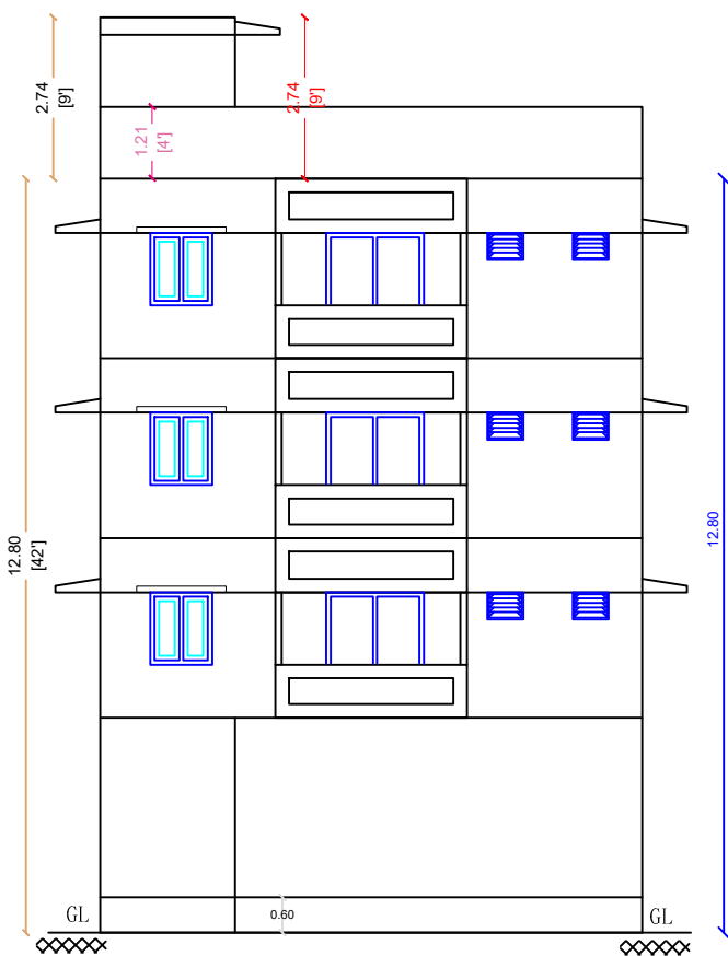
ELEVATION
