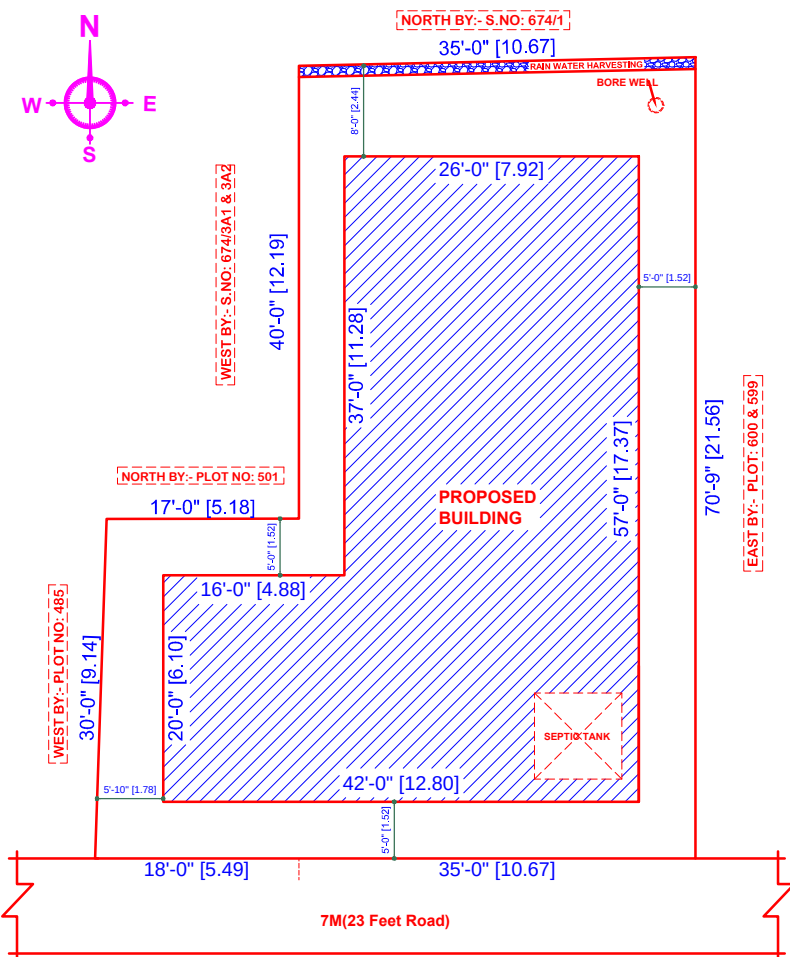
SITE PLAN (1:200)
