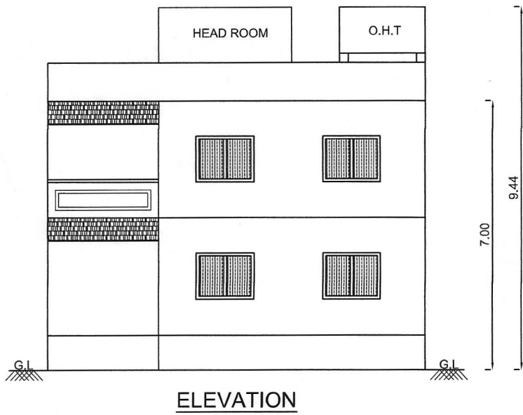
ELEVATION
