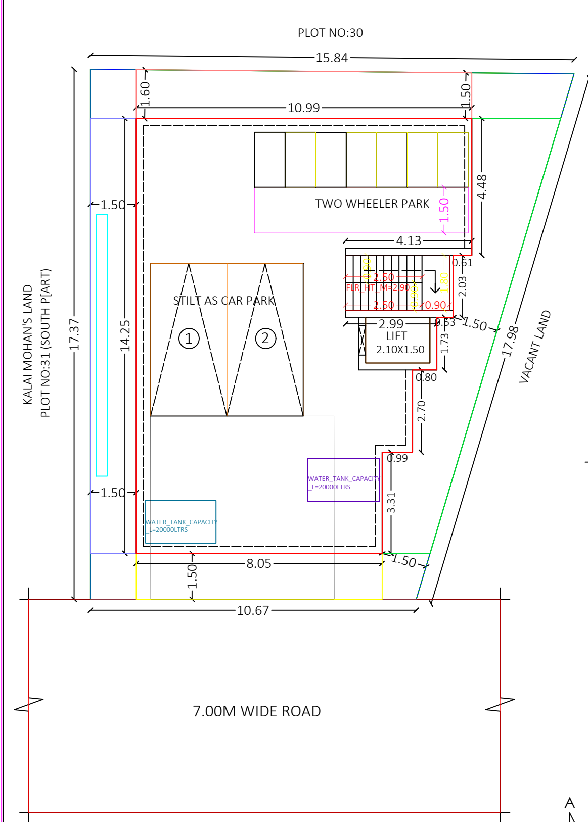
STLT CUM SITE PLAN
