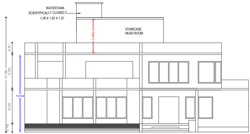
ELEVATION
