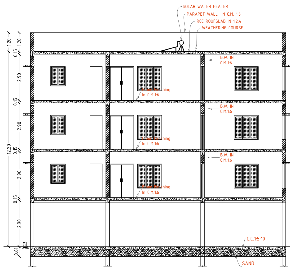
SECTION - A-A
