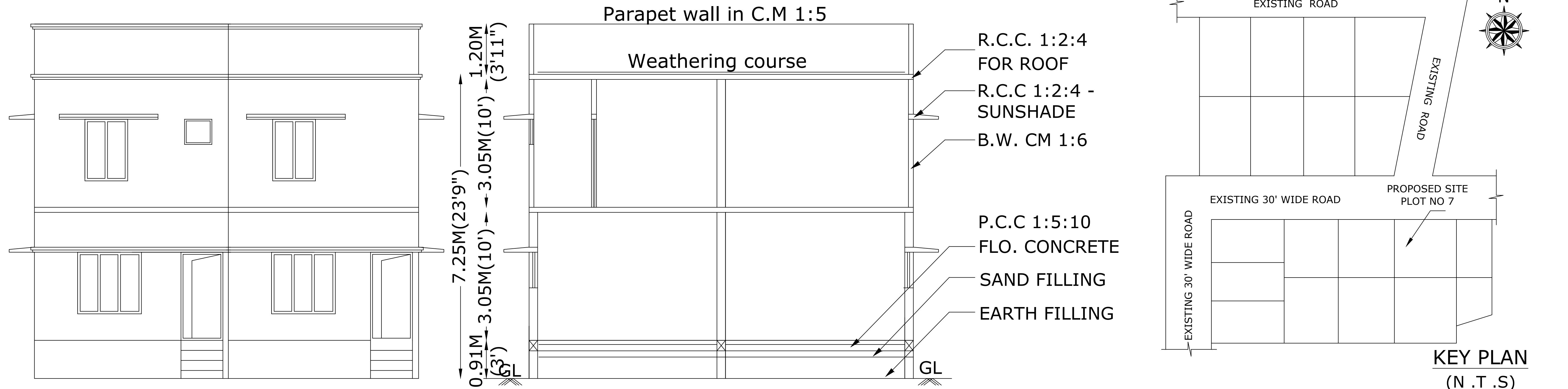
ELEVATION
