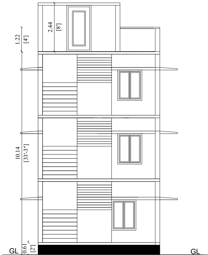
ELEVATION
