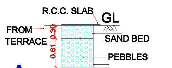
DETAILS OF R.W.H. TANK
