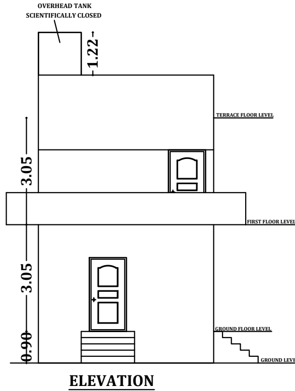
ELEVATION
