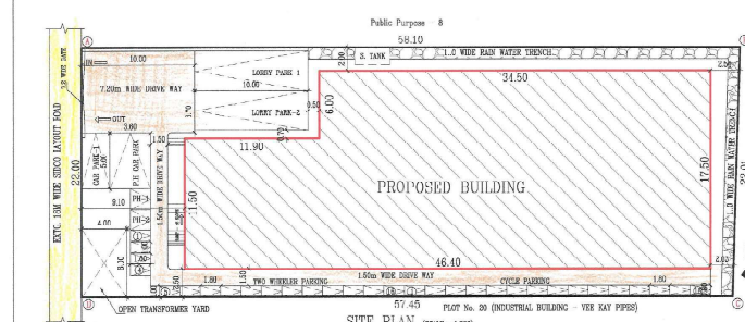
SITE PLAN (SCALE - 1:500)
