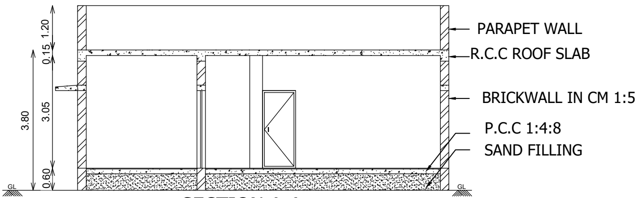
SECTION A-A
