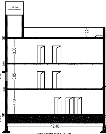
SECTION A-B
