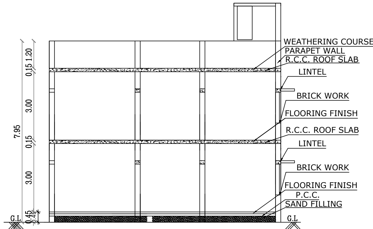
SECTION A-B
