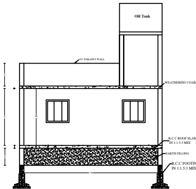
SECTION A-B
