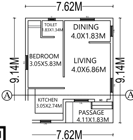
UND FLOOR PLAN
