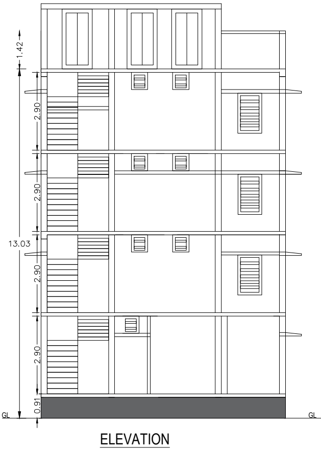
ELEVATION
