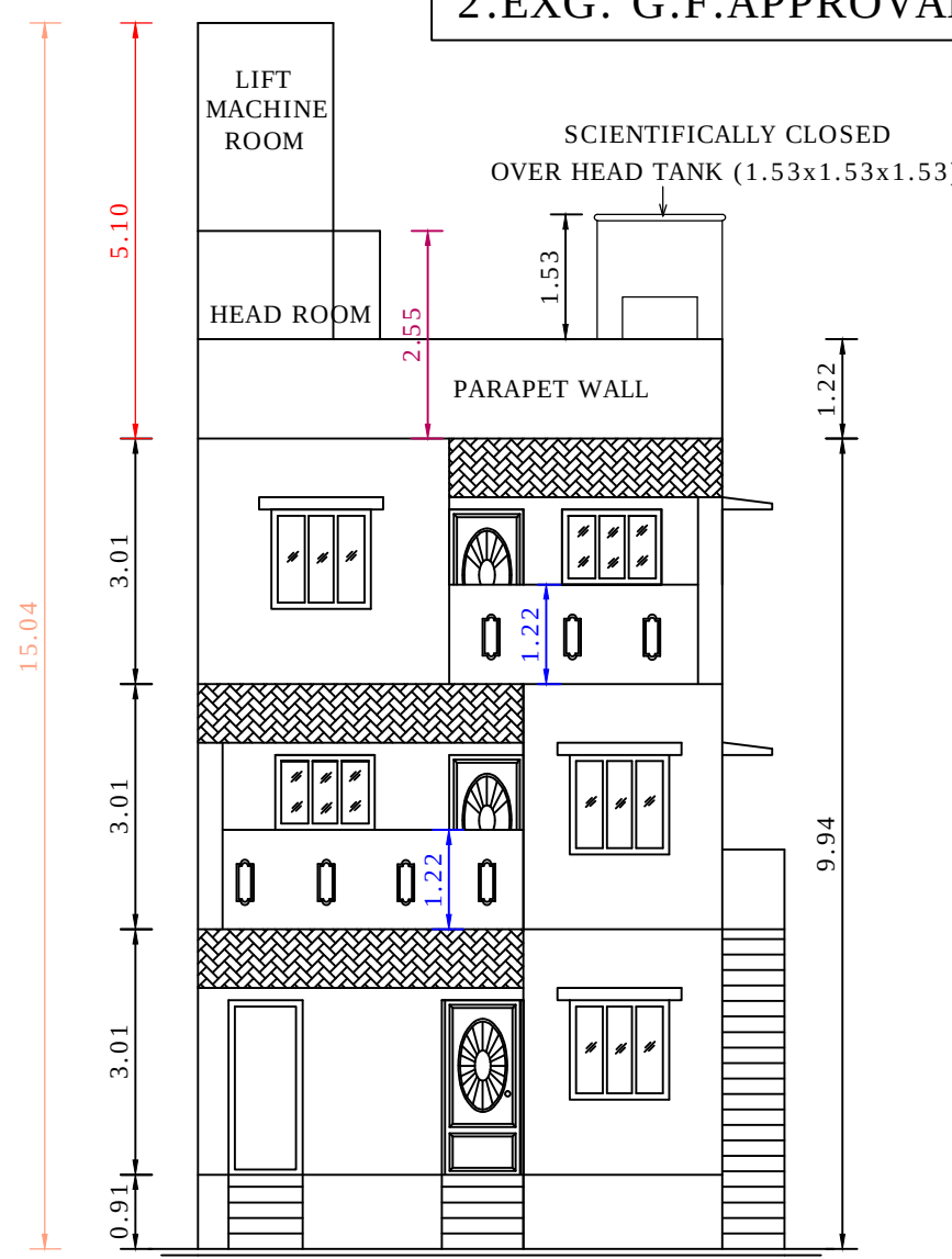
ELEVATION
