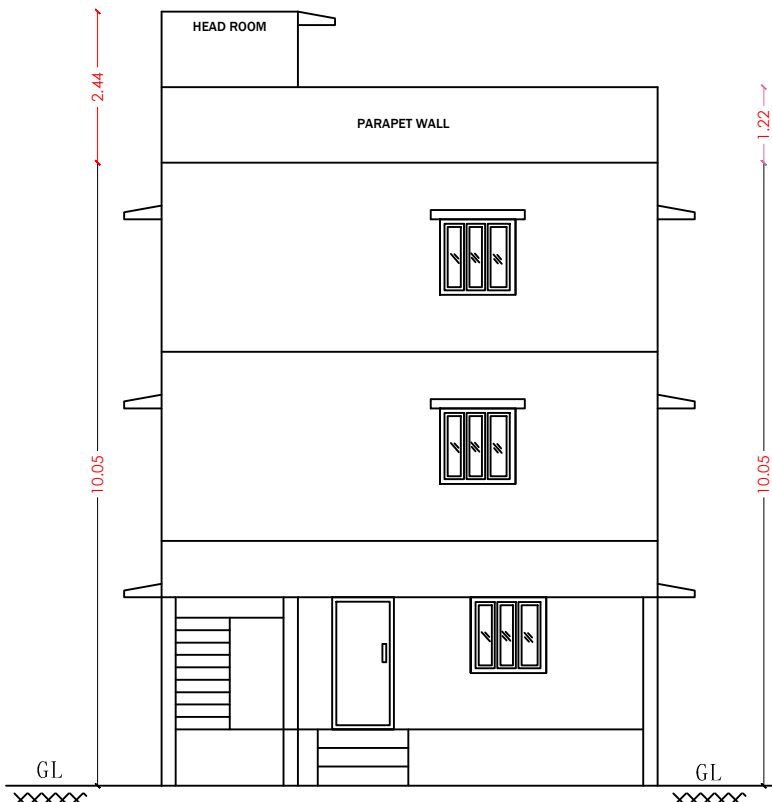
ELEVATION
