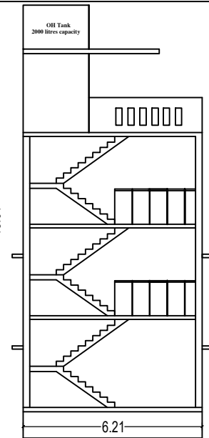
ELEVATION
