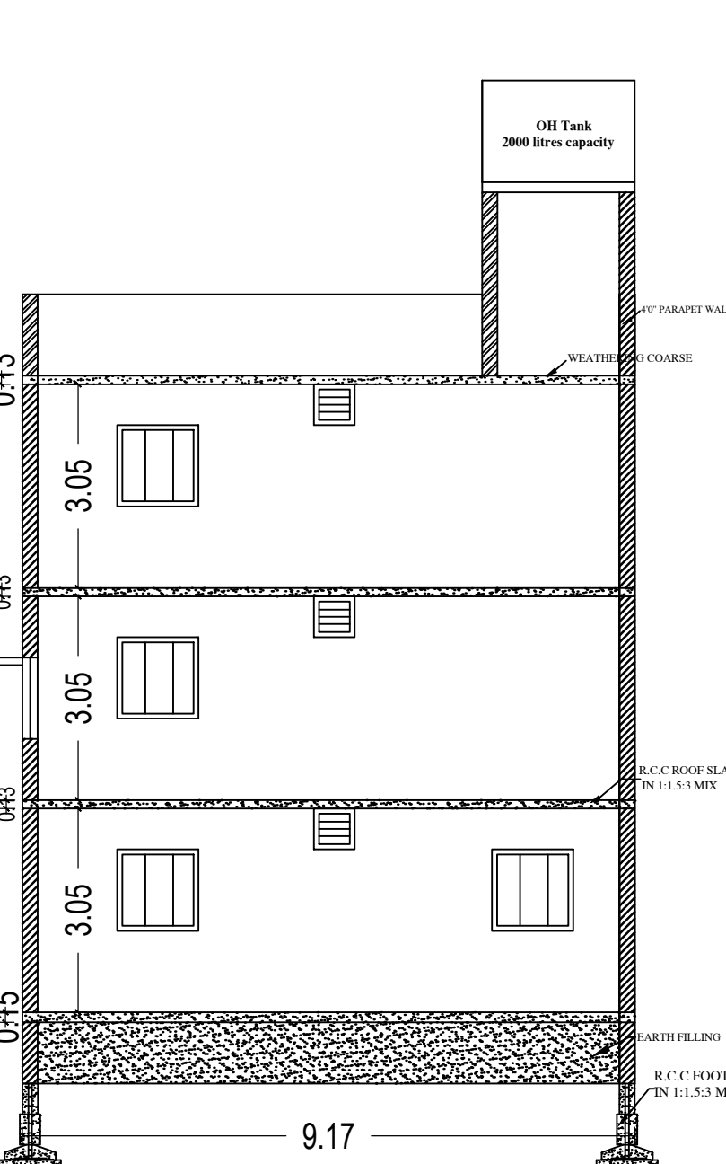
SECTION A-A
