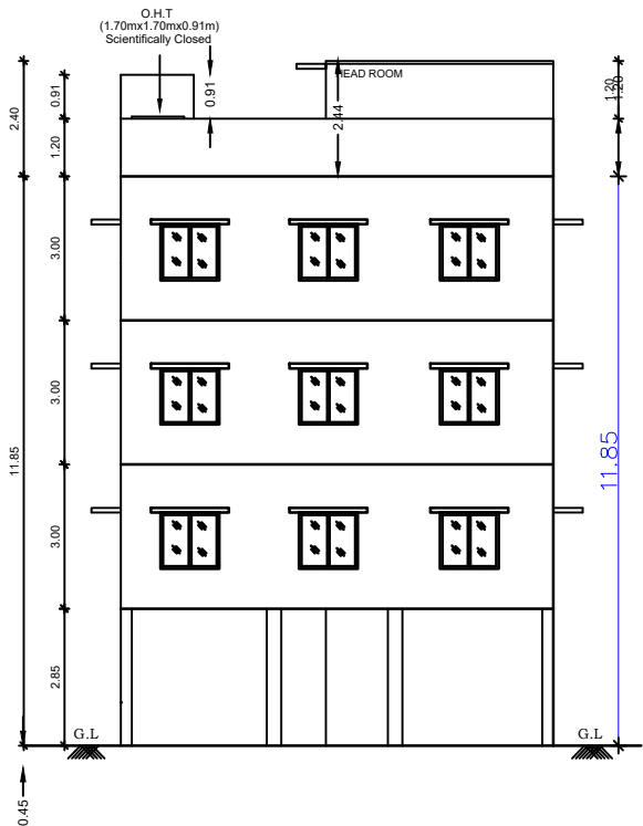
ELEVATION
