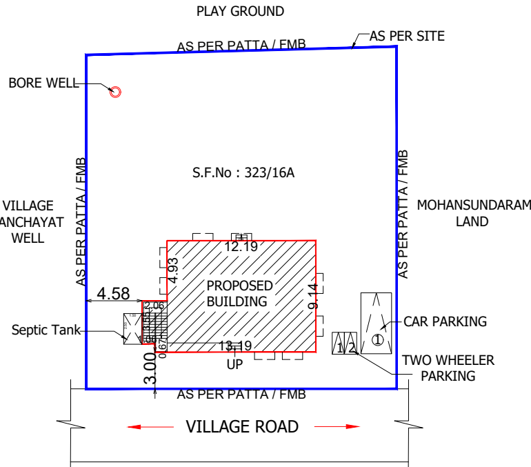
SITE PLAN SCALE 1:400
