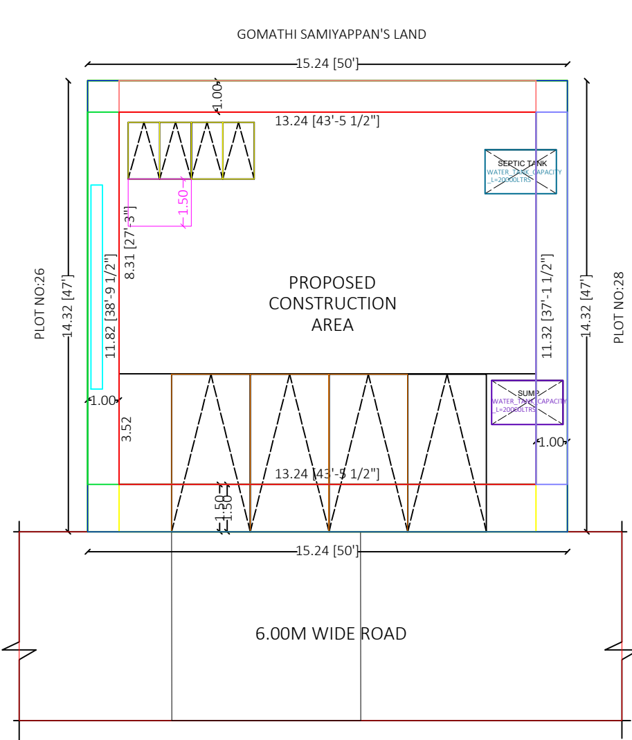
SITE PLAN SCLAE 1:100
