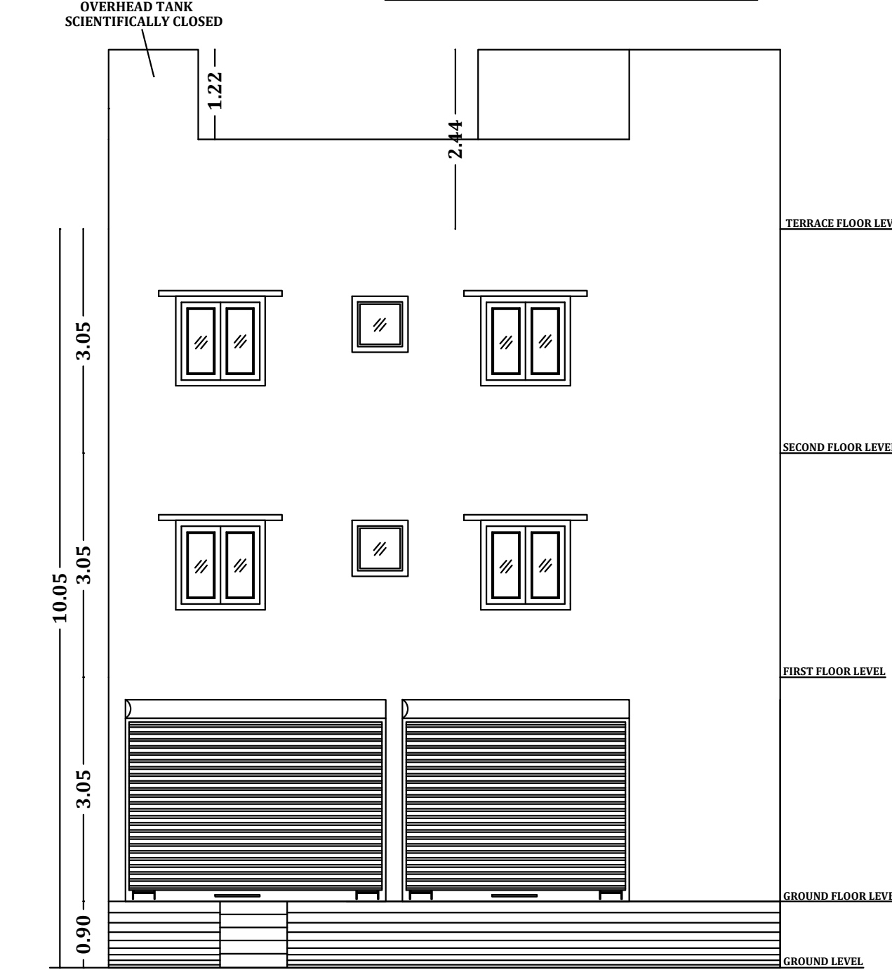
ELEVATION
