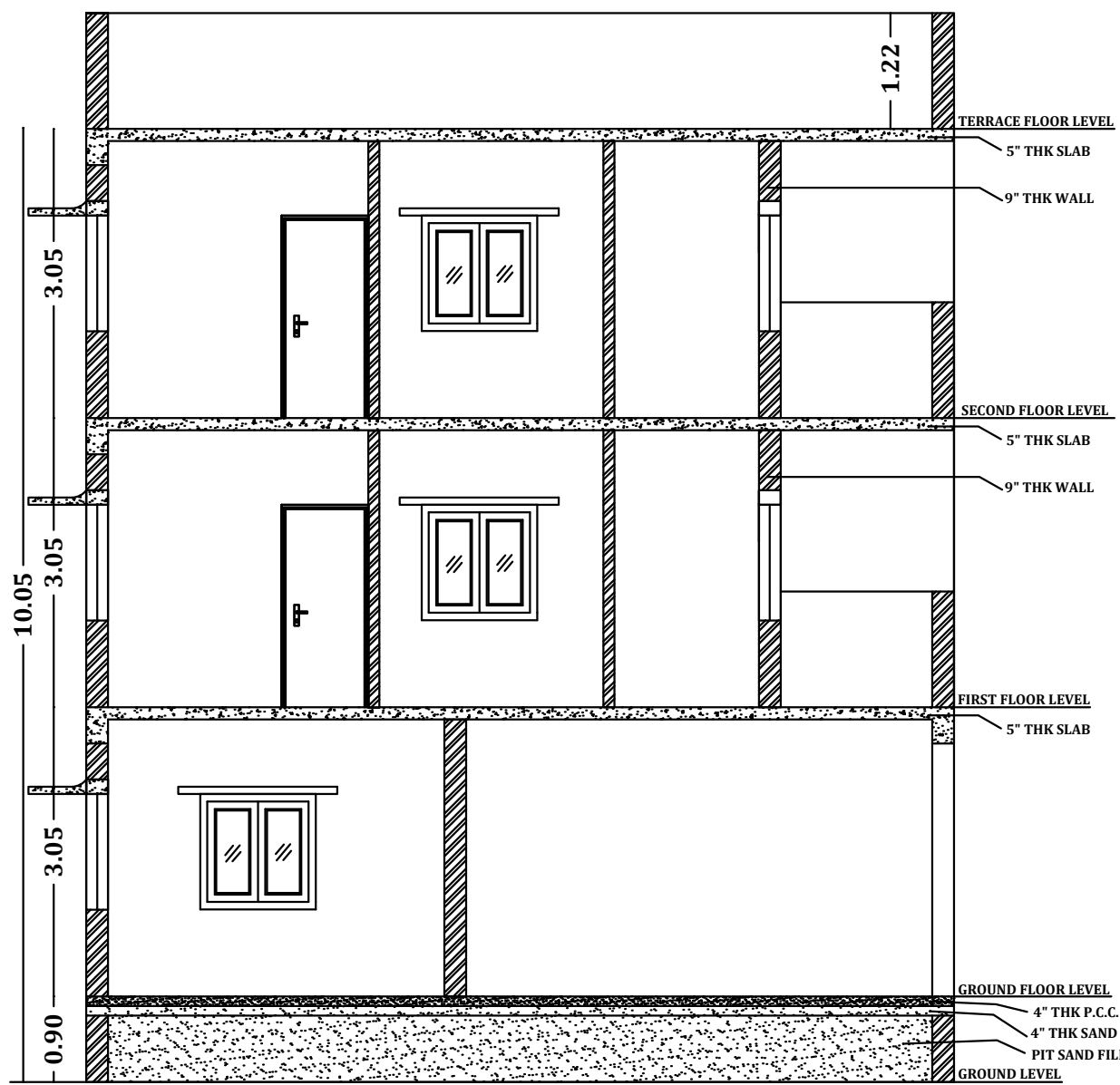
SECTION A-A'
