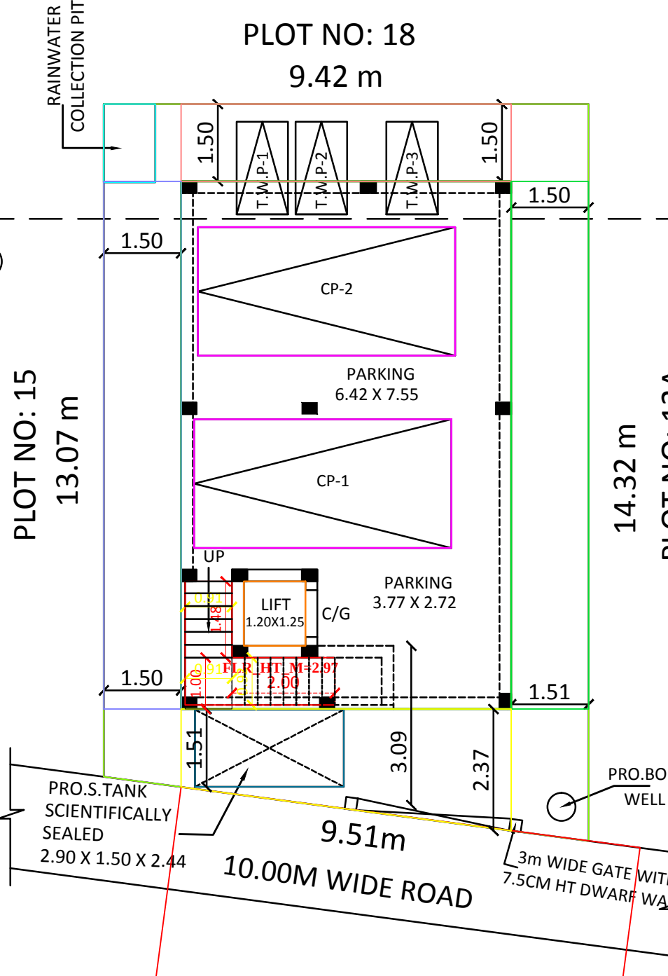
SITE CUM PRO. STILT FLOOR PLAN
