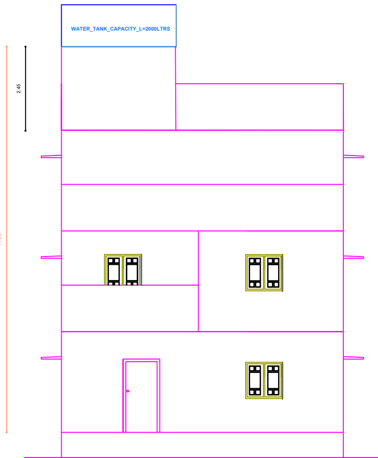
ELEVATION
