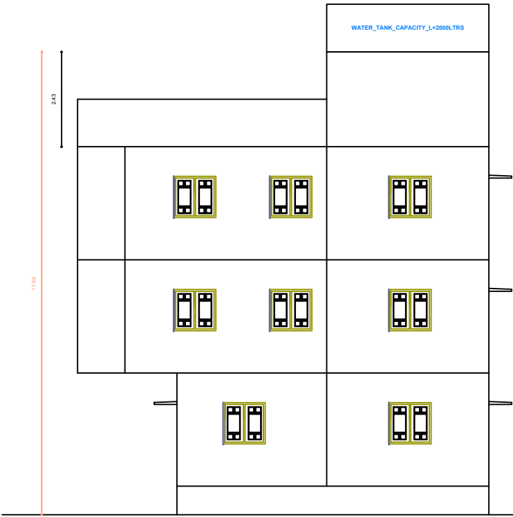
ELEVATION
