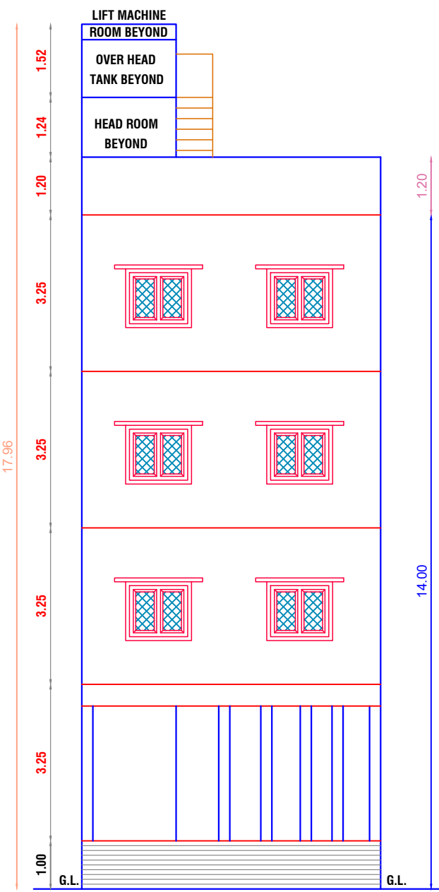
ELEVATION
