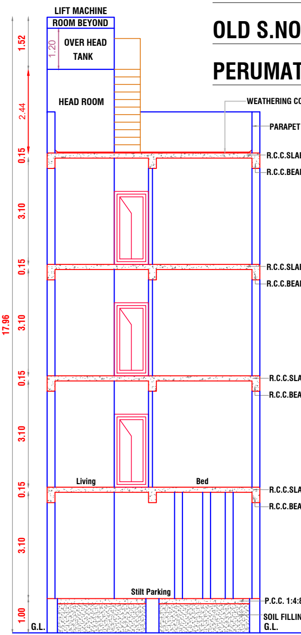
SECTION A-A
