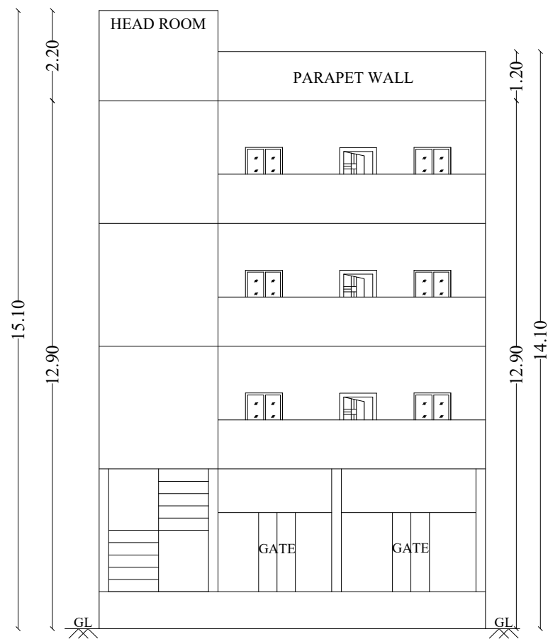
ELEVATION
