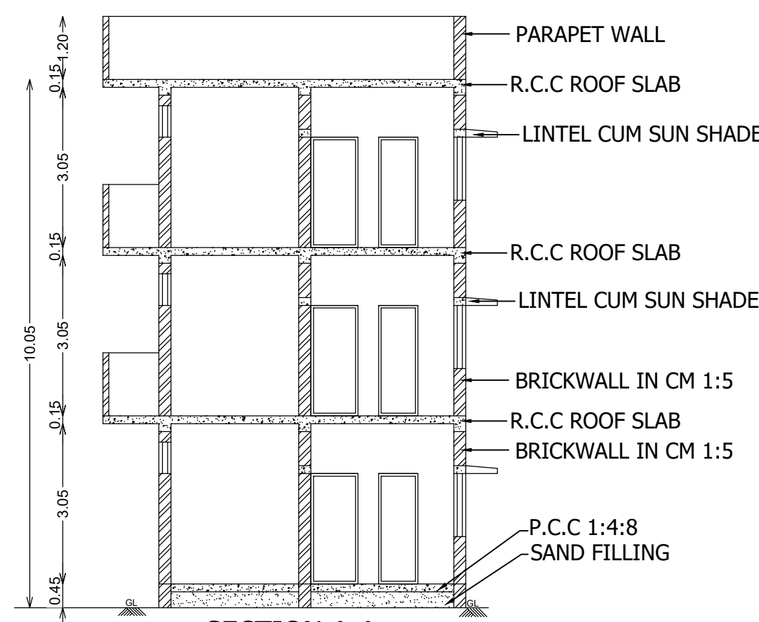
SECTION A-A
