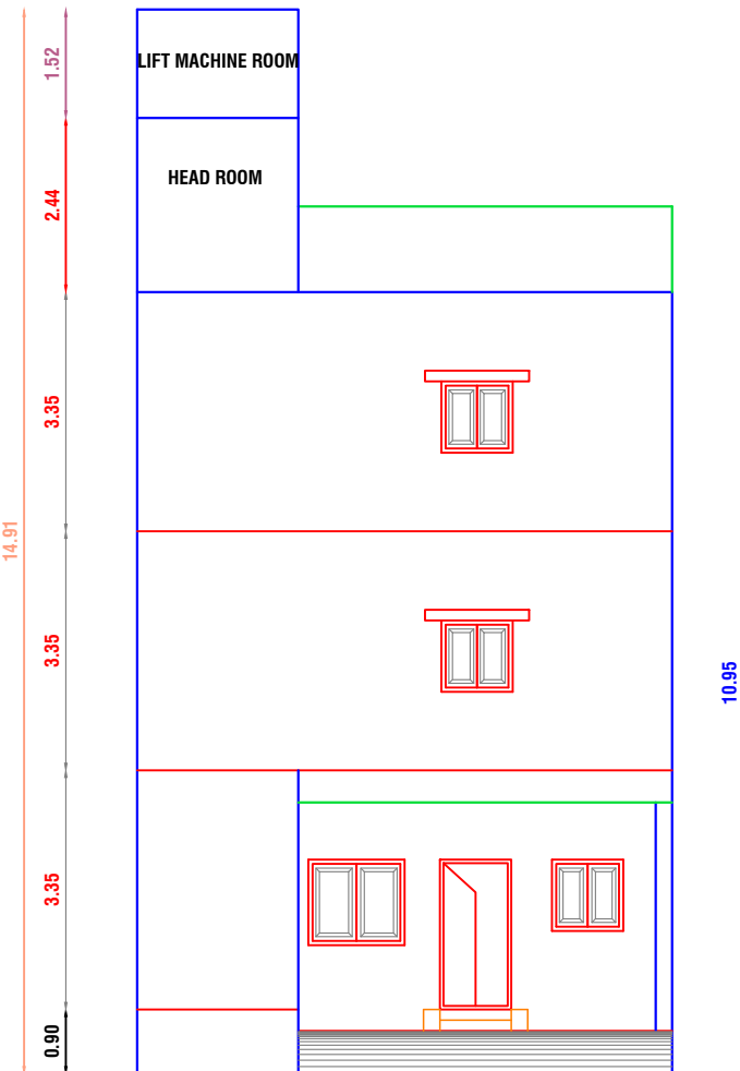
ELEVATION
