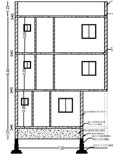
SECTION A-B
