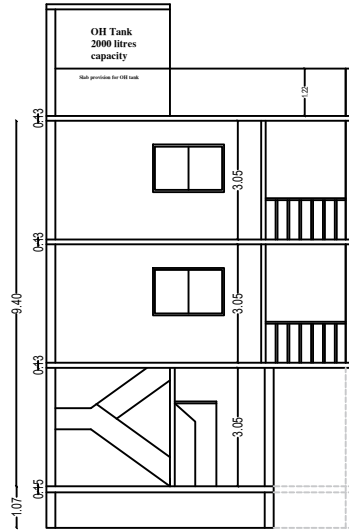
ELEVATION
