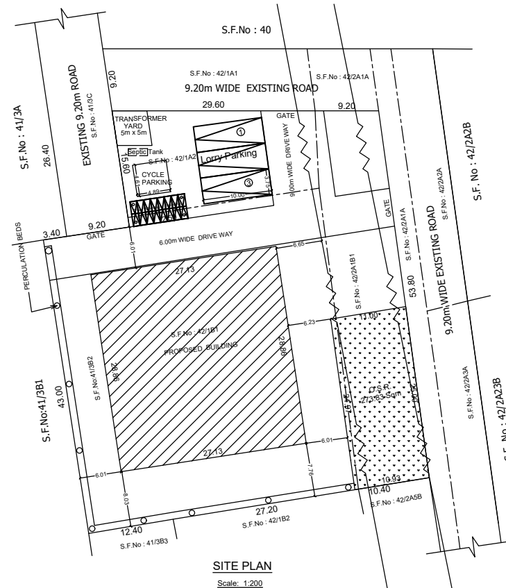
Scale: 1:200
