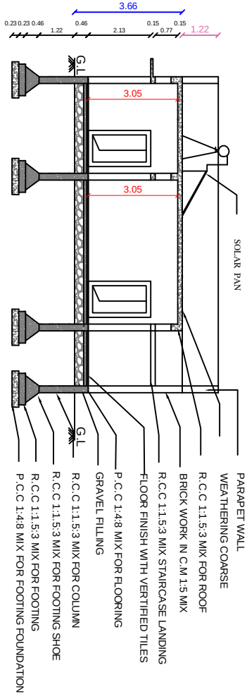
SECTION A-A'
