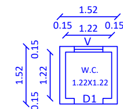
TOILET PLAN
