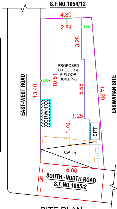
SITE PLAN 1:100
