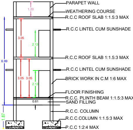
SECTION - AB
