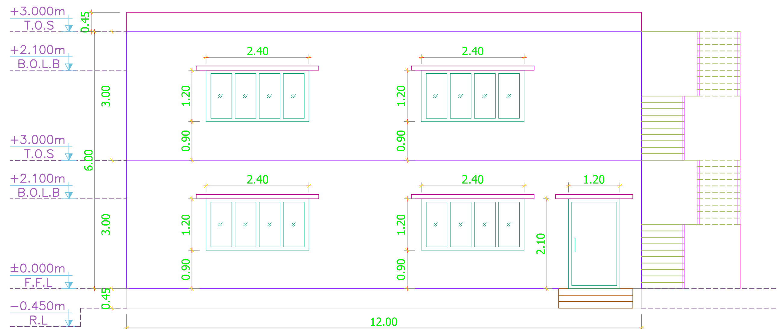
Elevation
