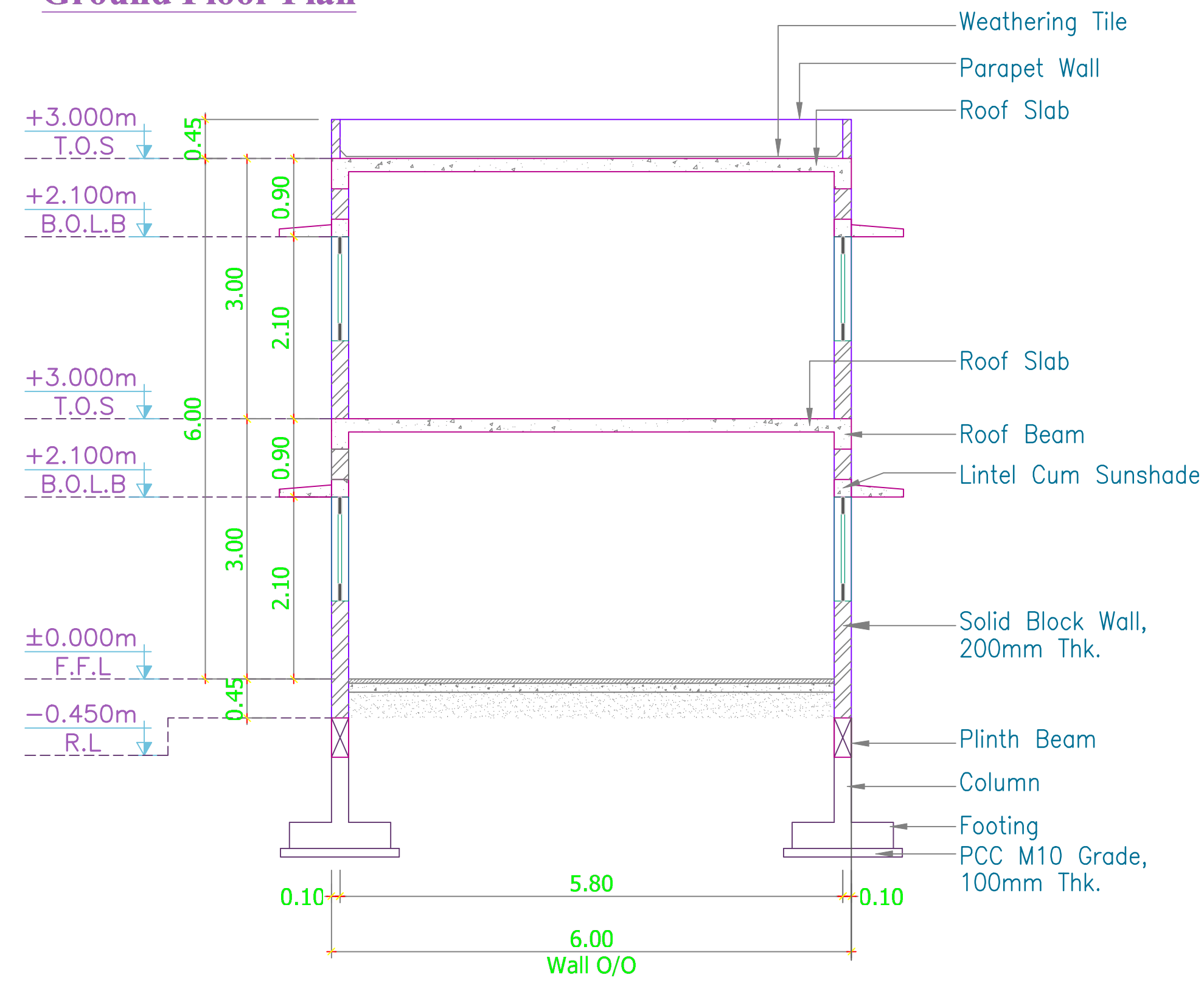
Section A-A
